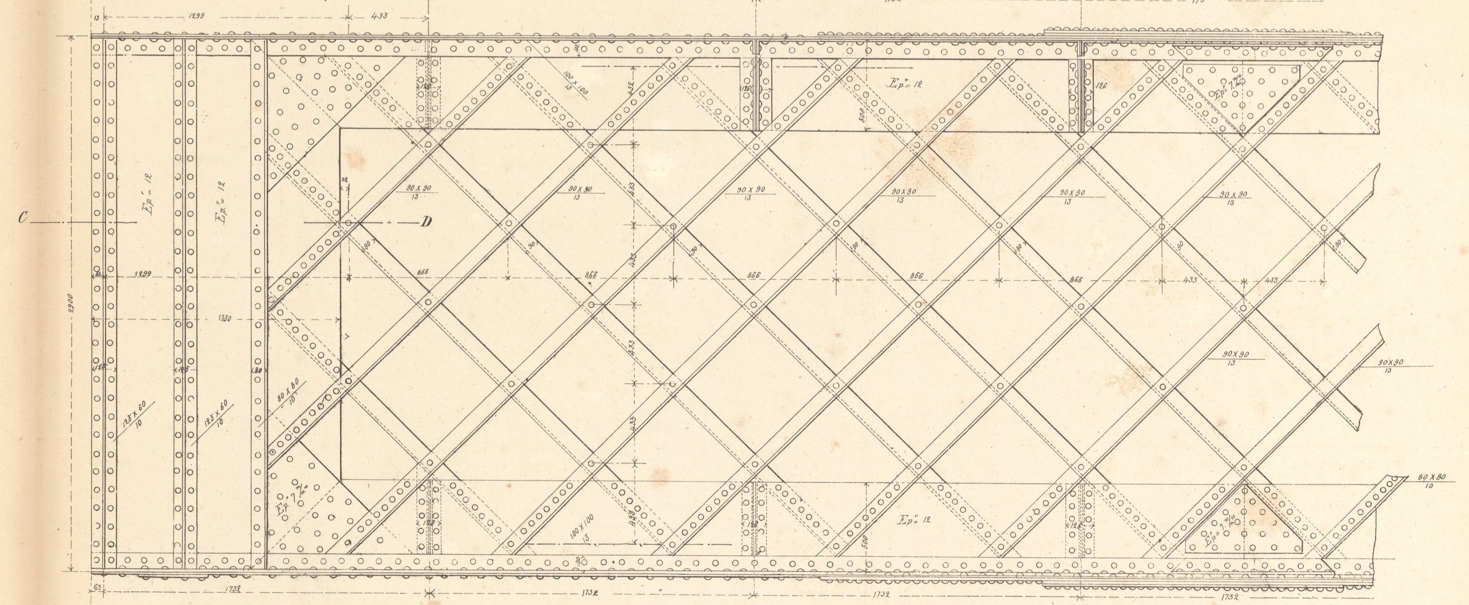
ELEVATION LONGITUDINALE D'UNE POUTRE PRINCIPALE (ab)
