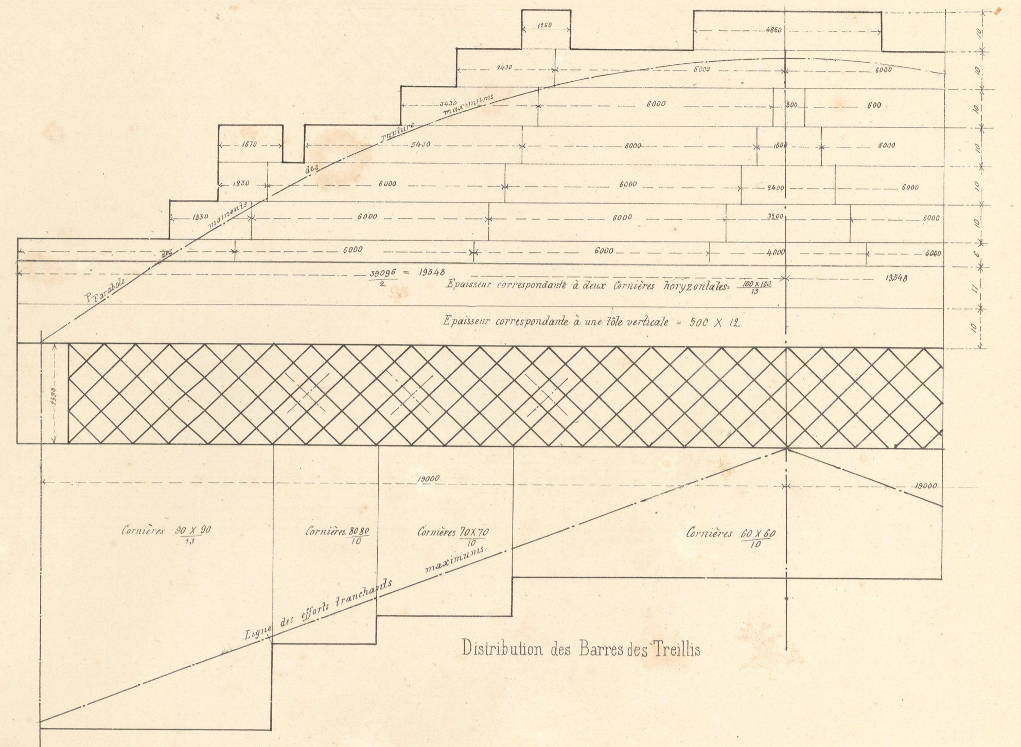
DISTRIBUTION DES TÔLES DES PLATEBANDES HORIZONTALES
