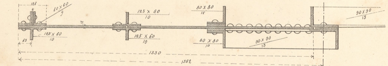
ELEVATION LONGITUDINALE D'UNE POUTRE PRINCIPALE (ab)
