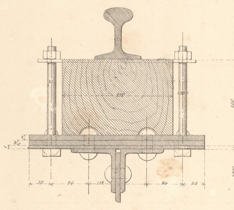
Attache des longhermes (b)
