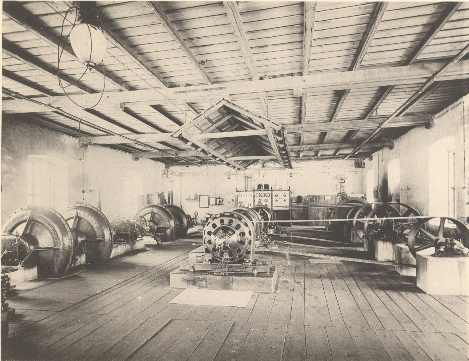
Maschinenhaus, Nordseite. Die Turbinen, Dynamos und Ventilatoren.
