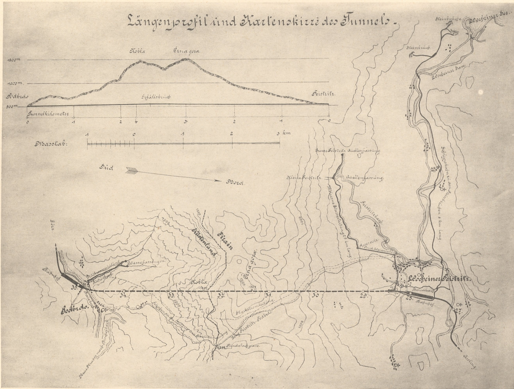
Längenprofil und Kartenskizze des Tunnels.
