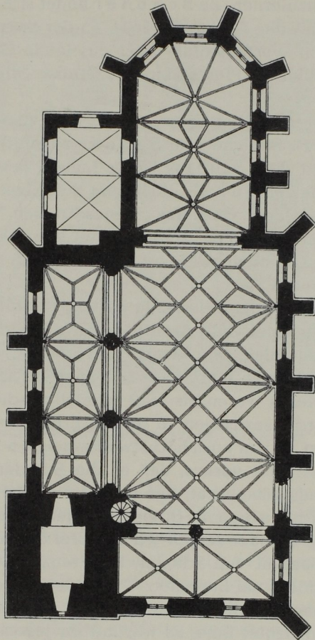
Abb. 268. Grundriß der Kirche Ranten.
