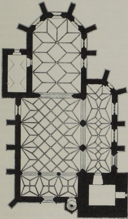
Abb. 267. Grundriß der Kirche Schöder.
