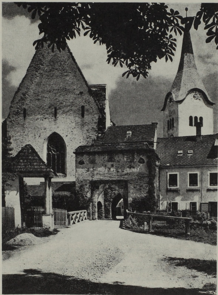
Abb. 245. Mittelalterliches Oberwölz.
