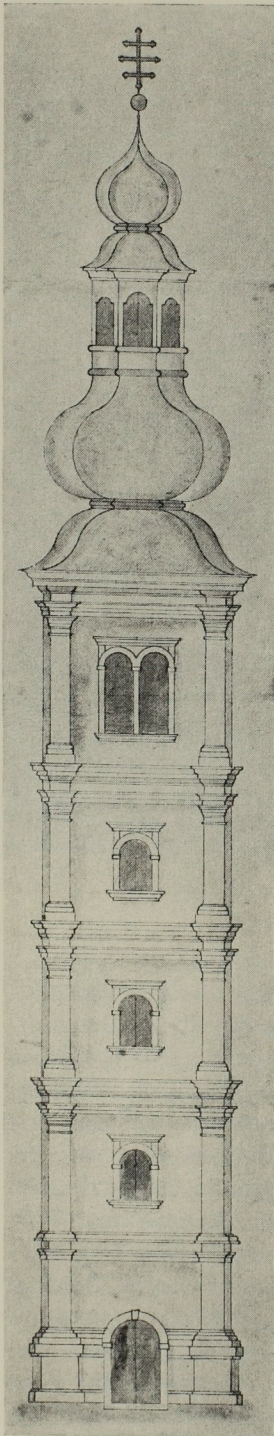
Abb. 222. Jakob Schmerlaib: Aufriß des Lankowitzer Kirch- turms.
