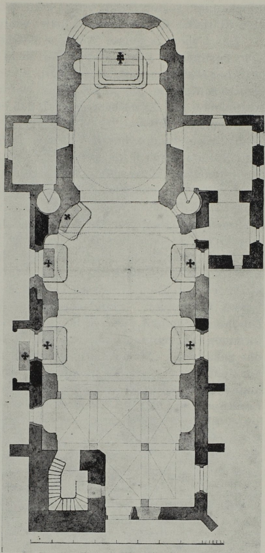
Abb. 205. Grundriß der Kindberger Pfarrkirche.
