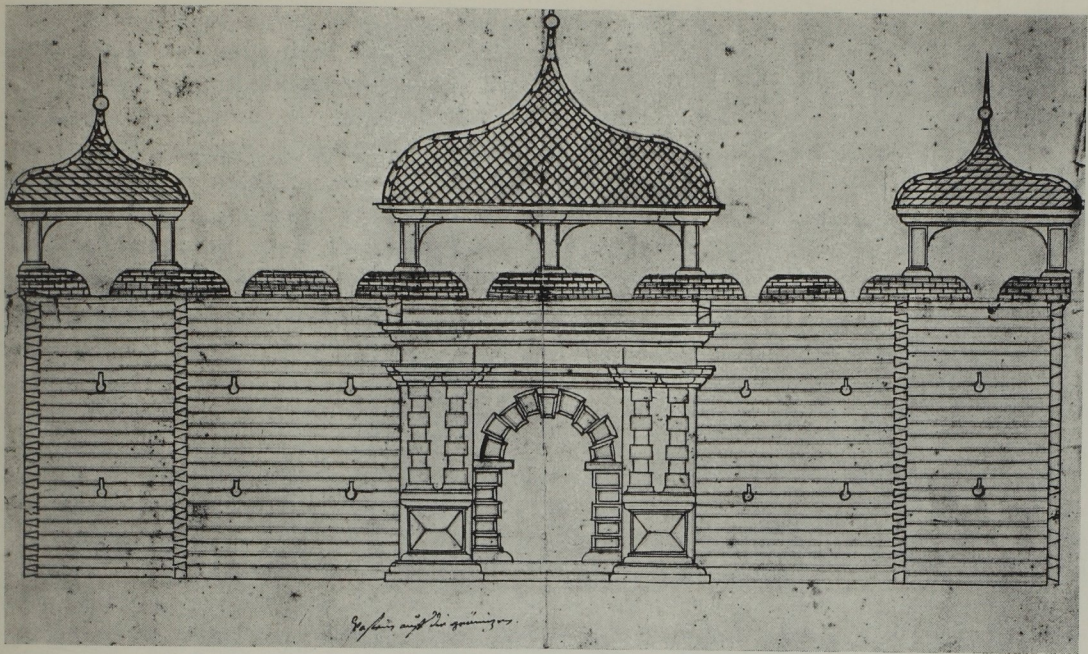
Abb. 102. Bauriß einer „Grenzbastei“. Zeichner und Bestimmungsort unbekannt
