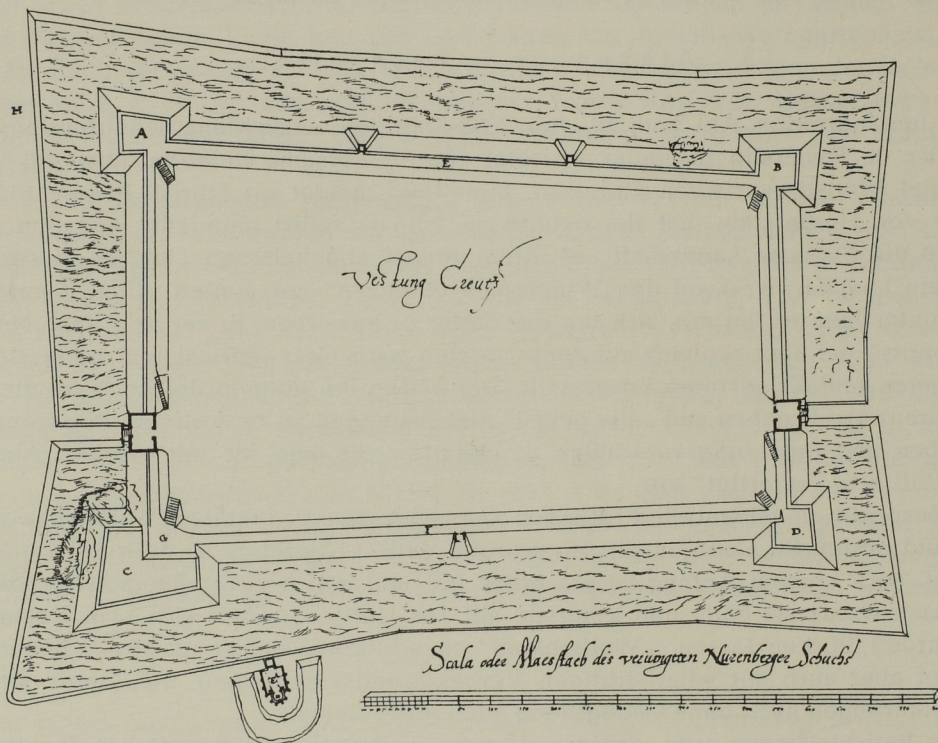
Abb. 43. Riß der Festung Kreuz von Alexander Pasqualini.
