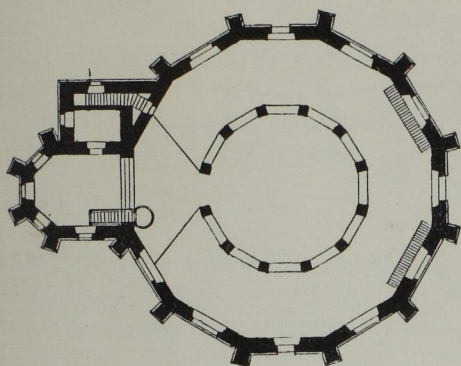
Abb. 83. Grundriß der Kirche
