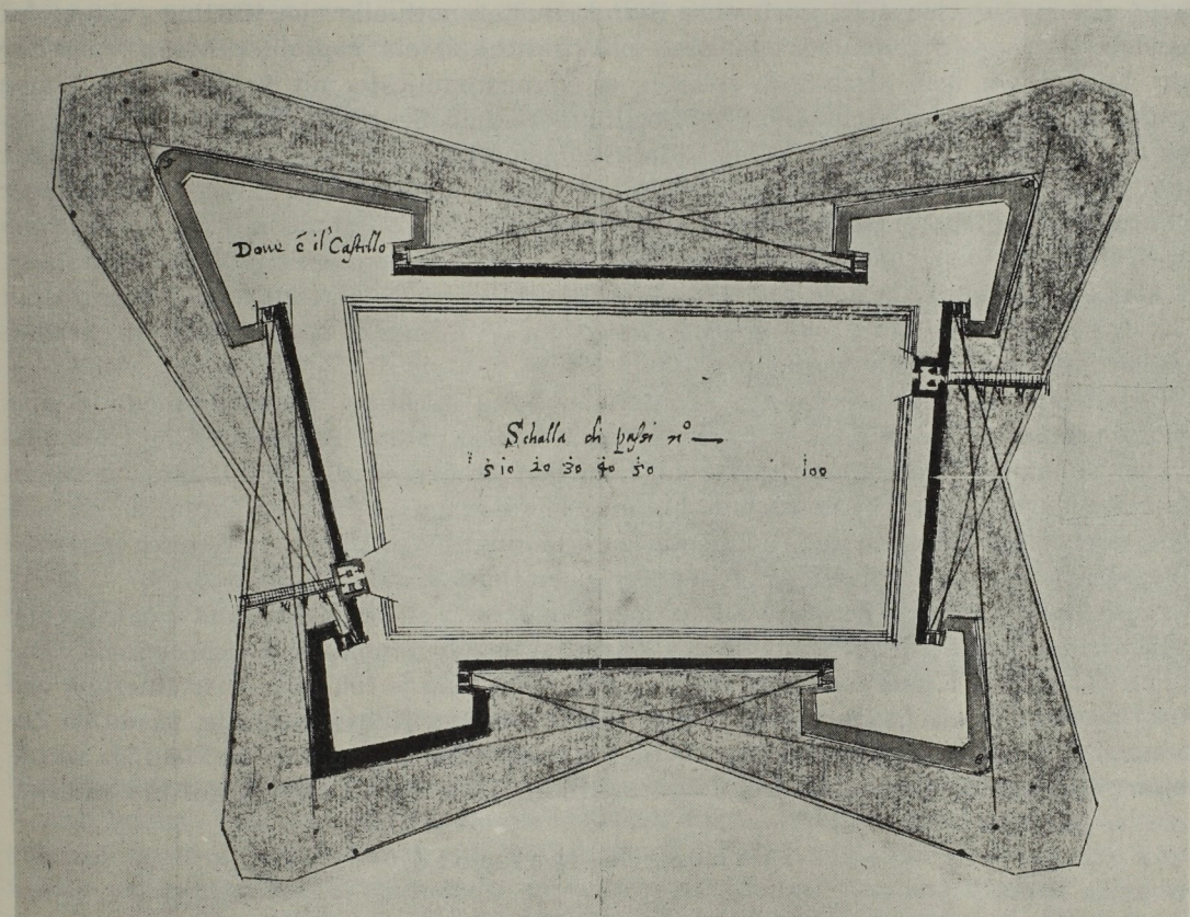
Abb. 41. Joseph Vintano: Festungsplan Copreiniz. 1582
