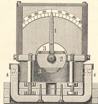
Fig. 1297. Galvanoskop.
