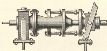
Fig. 1109. Schiebersteuerung.
