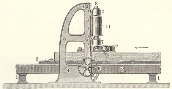
Fig. 644. Querhobelmaschine.
