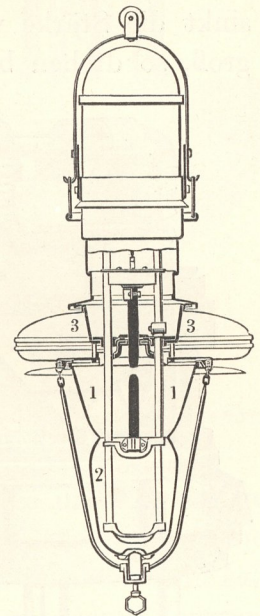
Fig. 477. Dauerbrand-Flammenbogenlampe der Allgemeinen Elektrizitäts-Gesellschaft.
