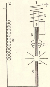
Fig. 476. Schema der Reginalampe.
