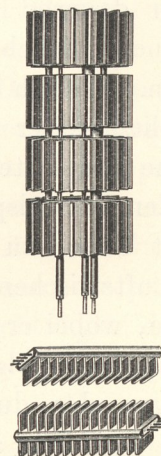
Fig. 439. Heizelemente elektrischer Öfen.
