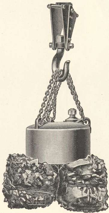
Fig. 440. Lastmagnet (Siemens-Schuckert-Werke).
