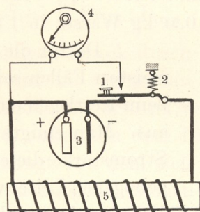
Fig. 306. Versuch zum Nachweis der Selbstinduktion.
