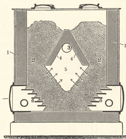
Fig. 211. Treppenrostgenerator.
