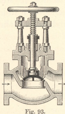
Fig. 93. Dampfabsperrentil.
