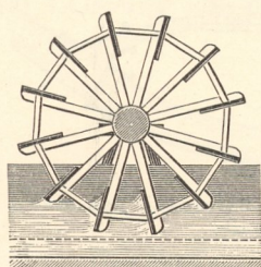
Fig. 24. Schiffmühlenrad.
