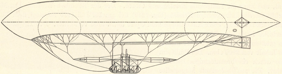
Fig. 1244. Österreichisches Militärluftschiff.
