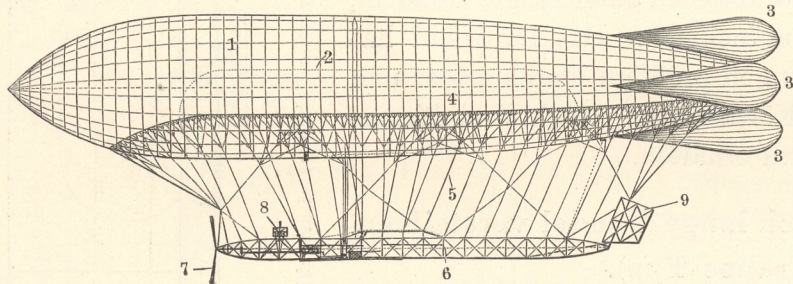
Fig. 1240. Luftschiff Clément Bayard I (1 Tragkörper, 2 Ballonet, 3 Dämpfungskörper, 4 Ballongurt, 5 Auslaufleinen, 6 Gondel, 7 Schraube, 8 Höhensteuer, 9 Seitensteuer).
