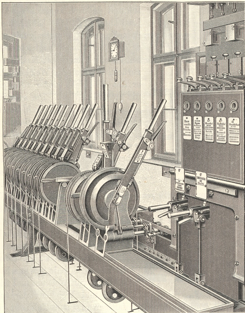
Fig. 1011. Stellwerk.
