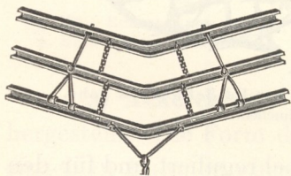
Fig. 794. Hoffmannsche Ackerschleife von W. Löhnert.
