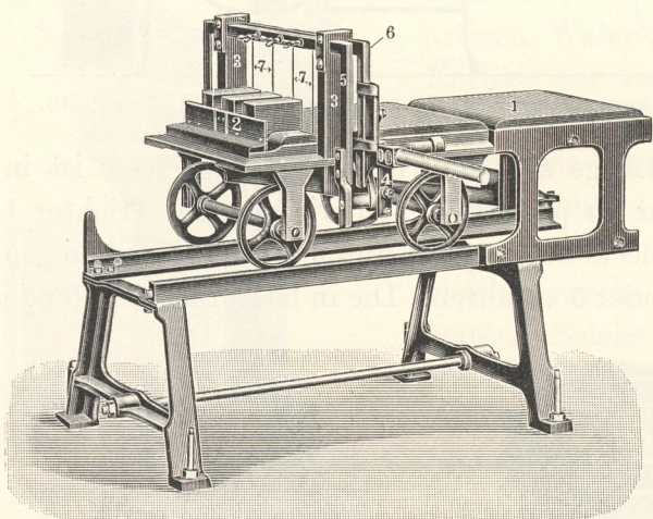
Fig. 625. Ziegel-Abschneideapparat.
