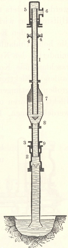
Fig. 573. Rittinger-Schacht- pumpe (Schnitt).
