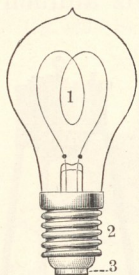
Fig. 488. Kohlenfadenlampe in Edisonfassung.
