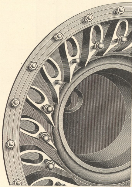
Fig. 51. Drehschaufeln, offen.
