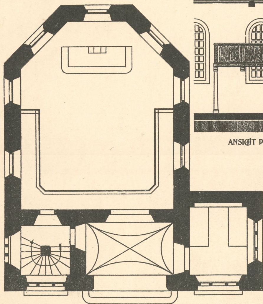
GRUNDRISS
