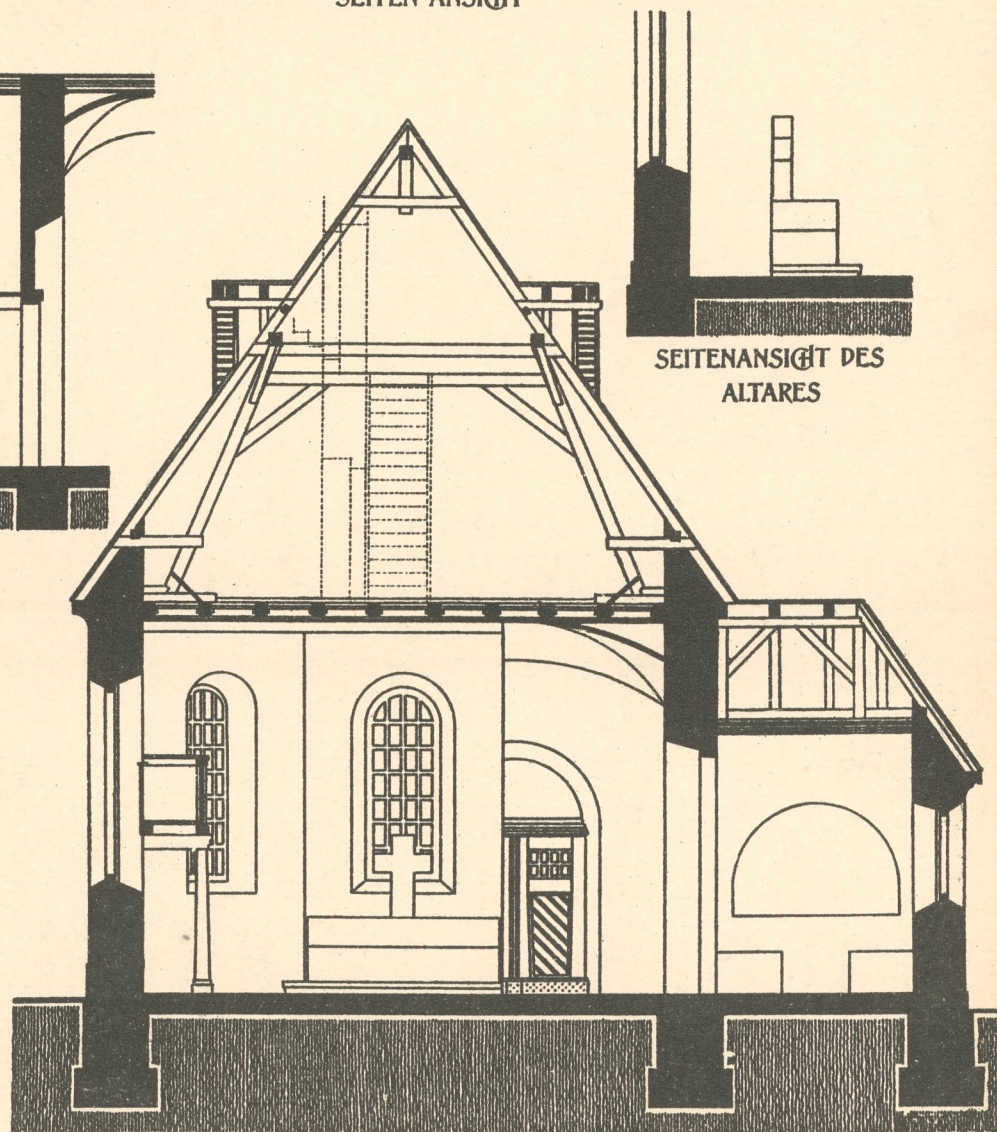
QUERSCHNITT
