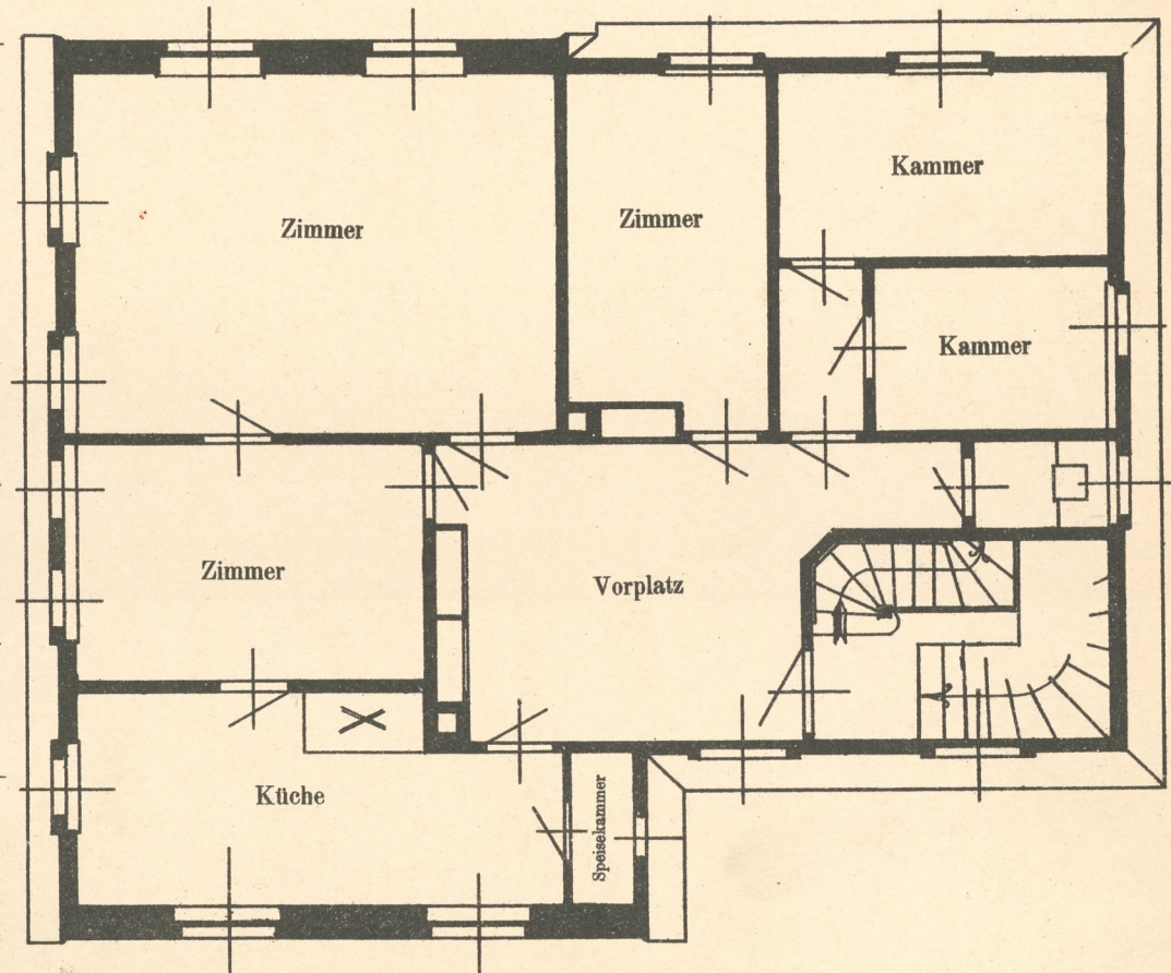
OBERGESCHOSS
