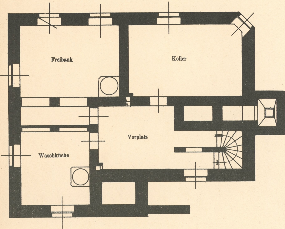
KELLERGESCHOSS
