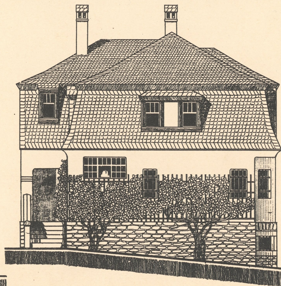
SEITENANSICHT
