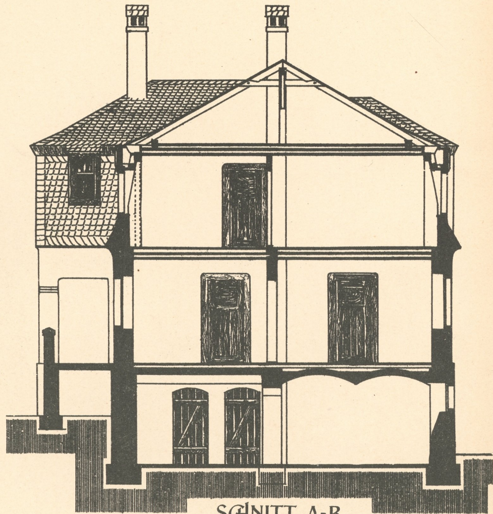
SCHNITT A-B
