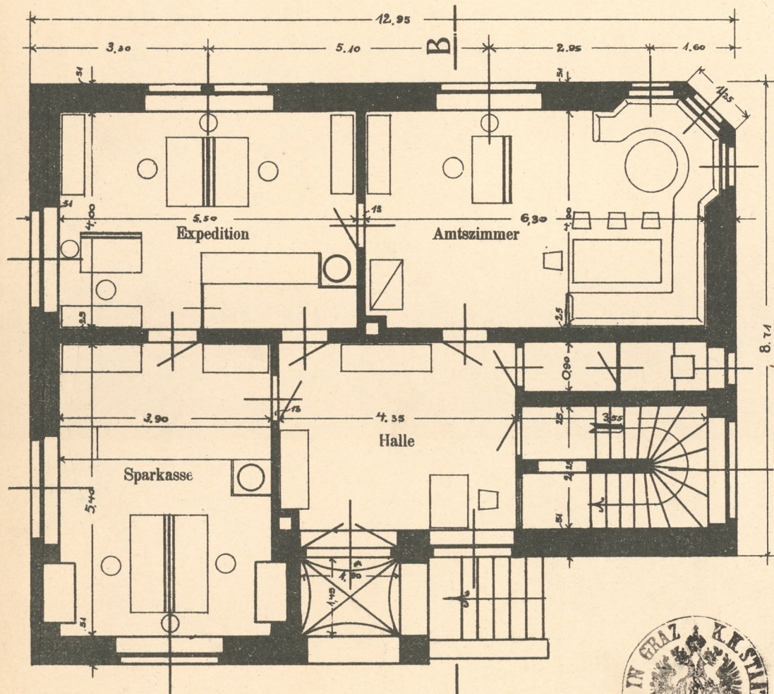
ERDGESCHOSS
