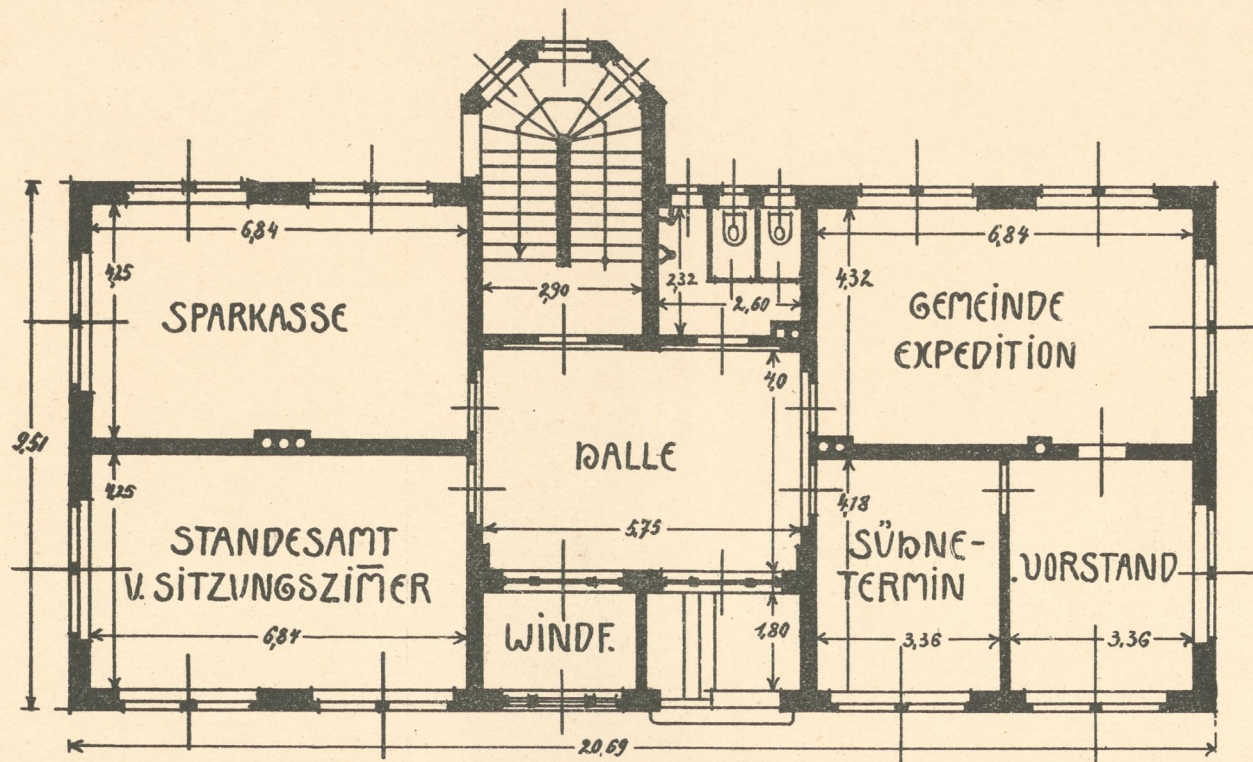
ERDGESCHOSS
