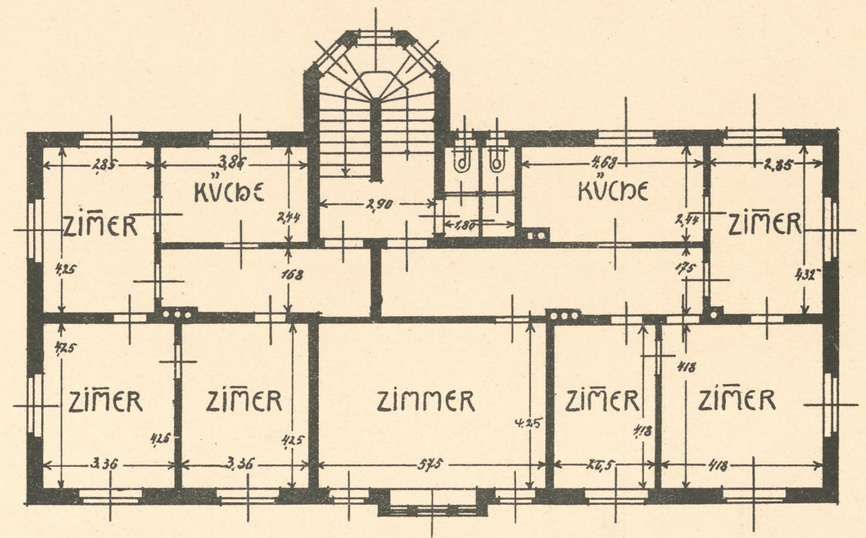
OBERGESCHOSS
