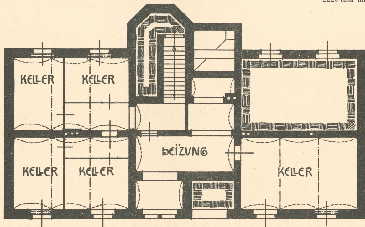
KELLERGESCHOSS
