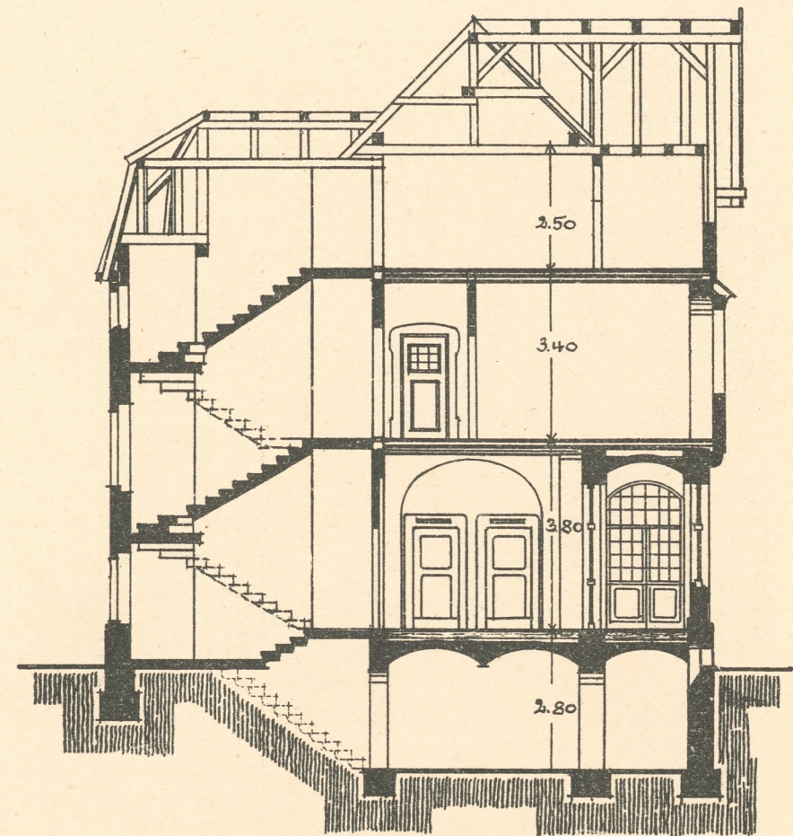
QUERSCHNITT
