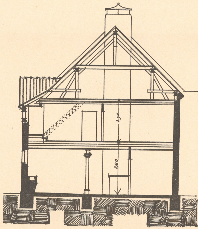
SCHNITT.
