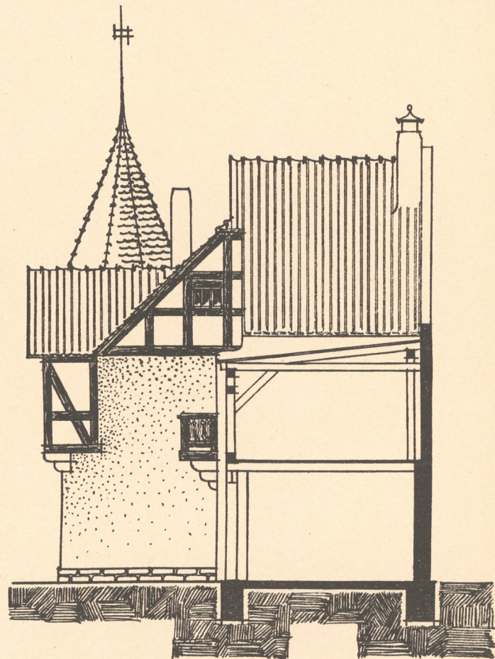
RECHTE GIEBELANSICHT.
