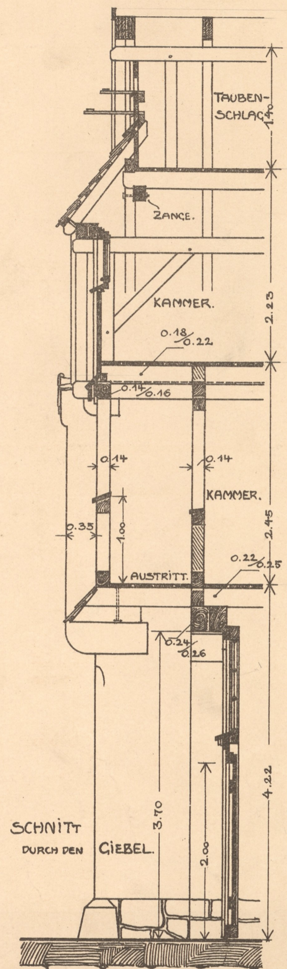
DETAILANSICHT VOM WOHNHAUSE DES MUSTERGEHÖFTES DER DEUTSCHEN BAUAUSSTELLUNG DRESDEN 1900.
