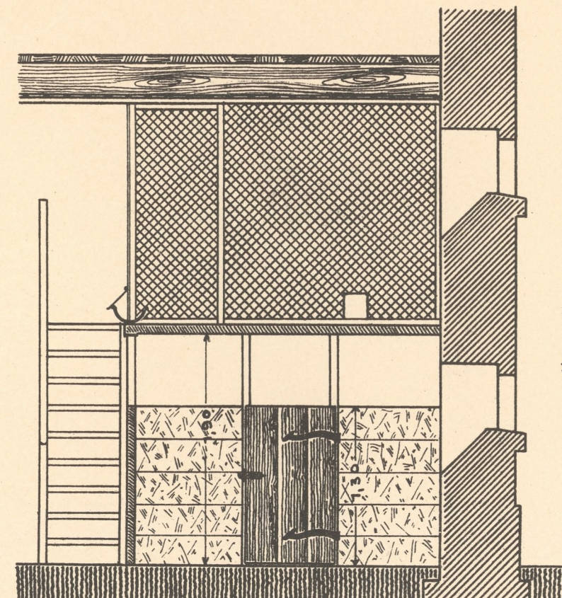
SCHNITT C-D
