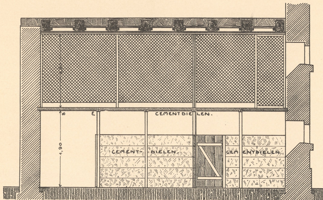
SCHNITT A-B
