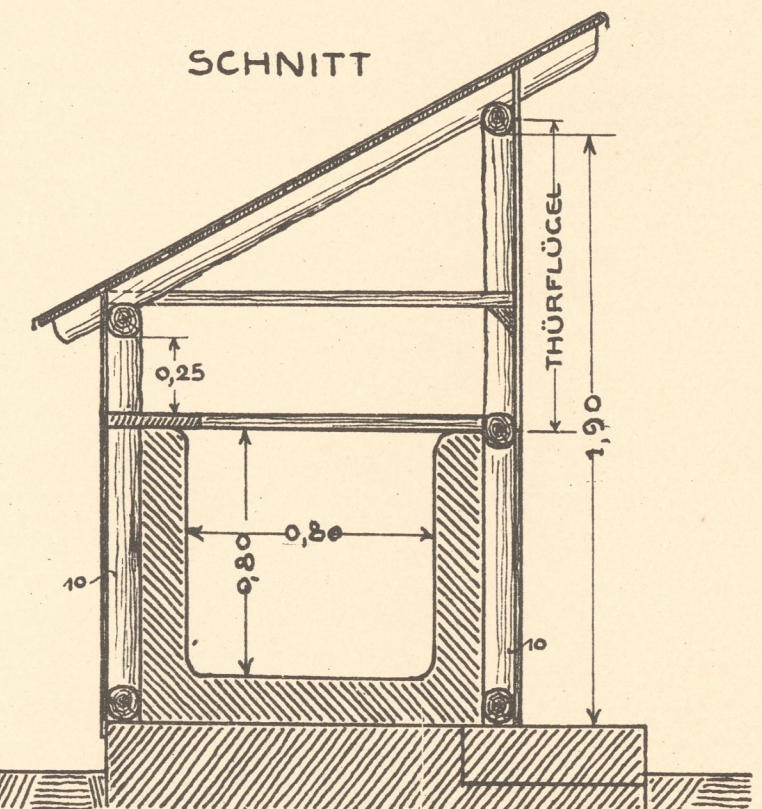
WASSERHÄUSCHEN.
