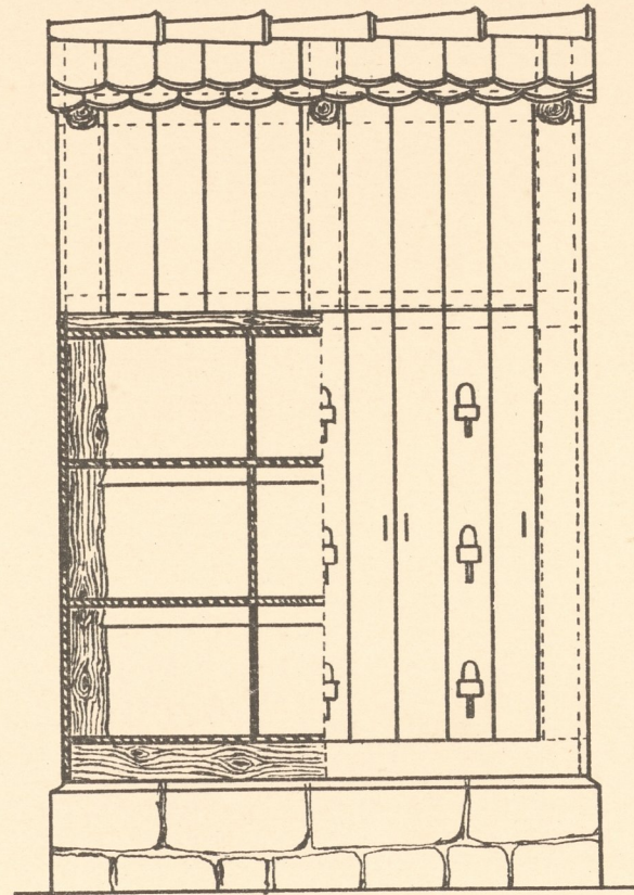
VORDERANSICHT.
