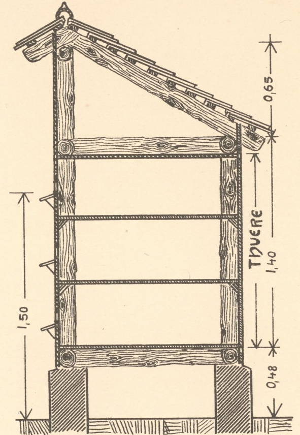
SCHNITT
