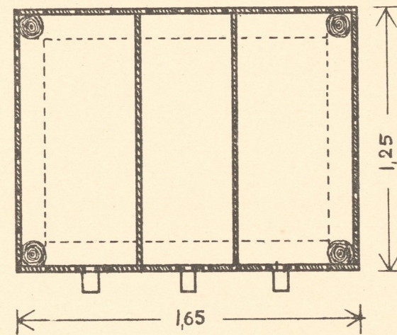
GRUNDRISS.
