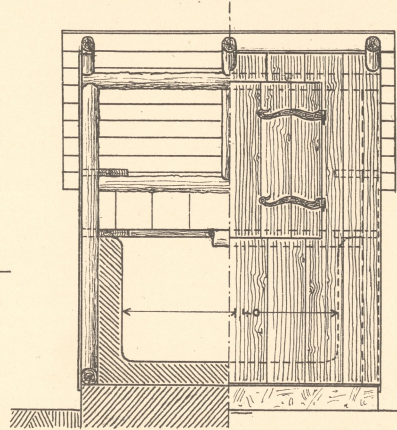
WASSERHÄUSCHEN.
