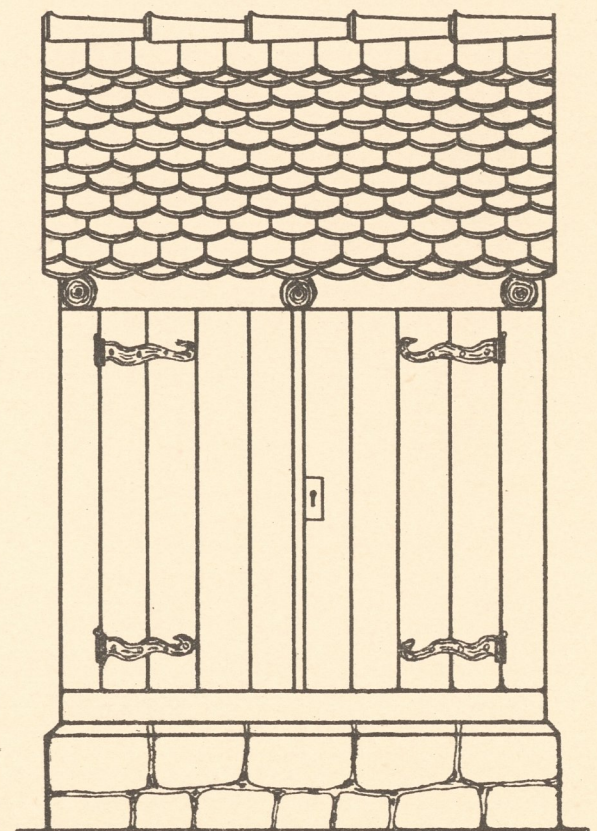
RÜCKANSICHT.
