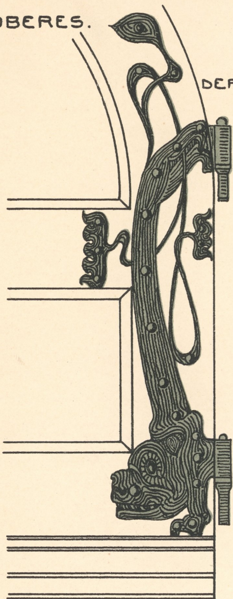
BESCHLÄGE DER ZWEIFLÜGLIGEN HAUSTHÜRE.
