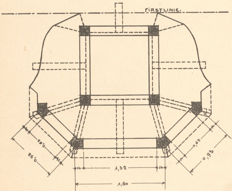
SCHNITT E-F
