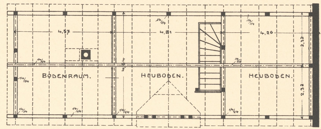
DACHGESCHOSS.
