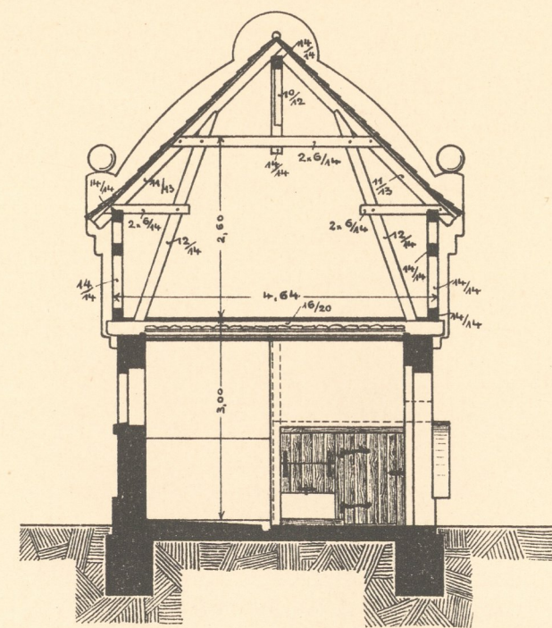
DACHGESCHOSS.
