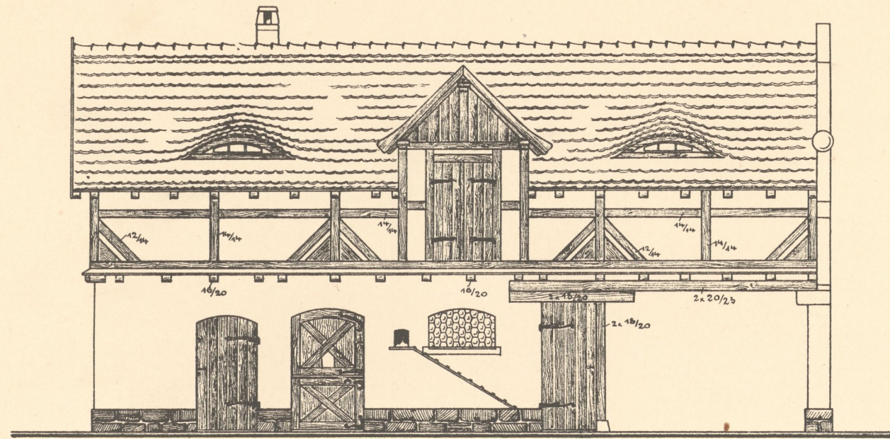
ANSICHT.
