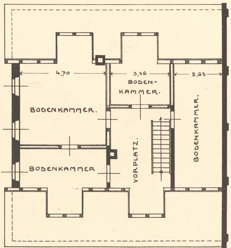
2. OBERGESCHOSS.
