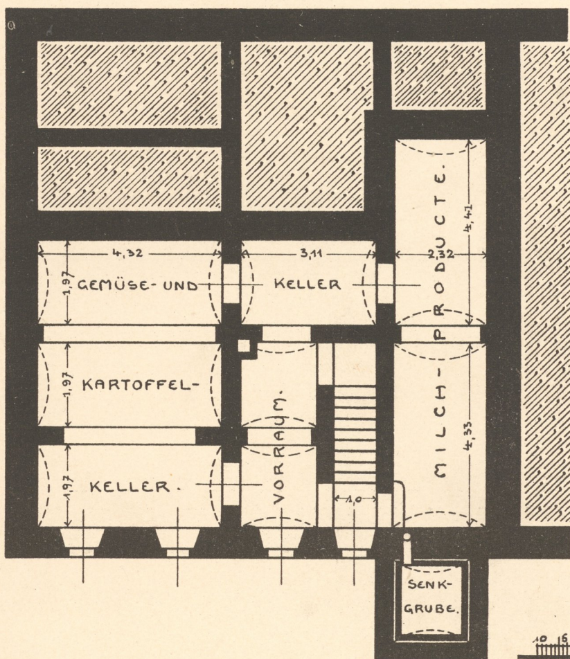
KELLERGESCHOSS
