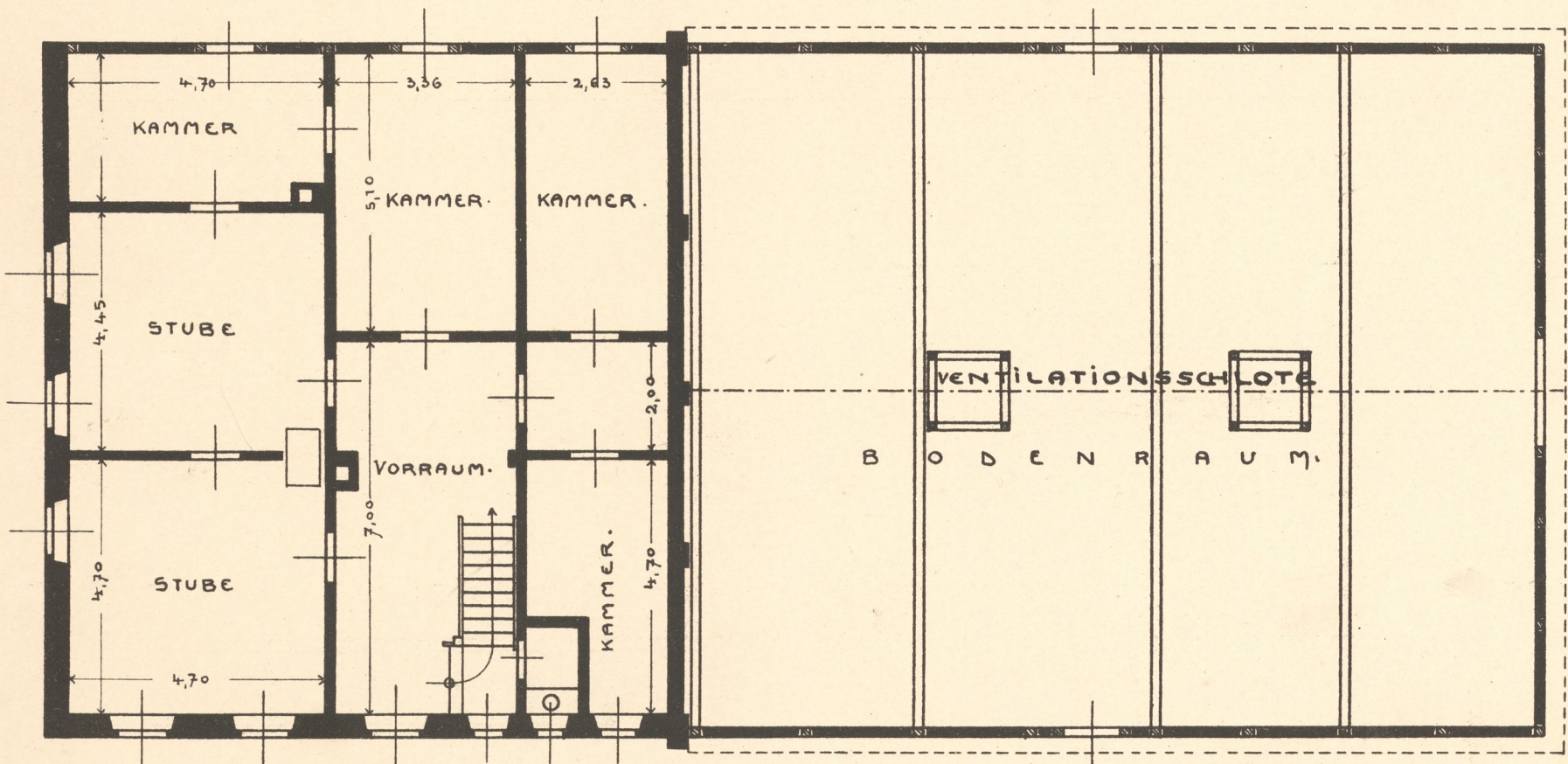
OBERGESCHOSS
