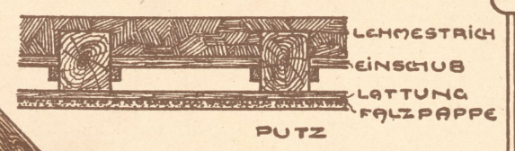
DECKENDETAIL
