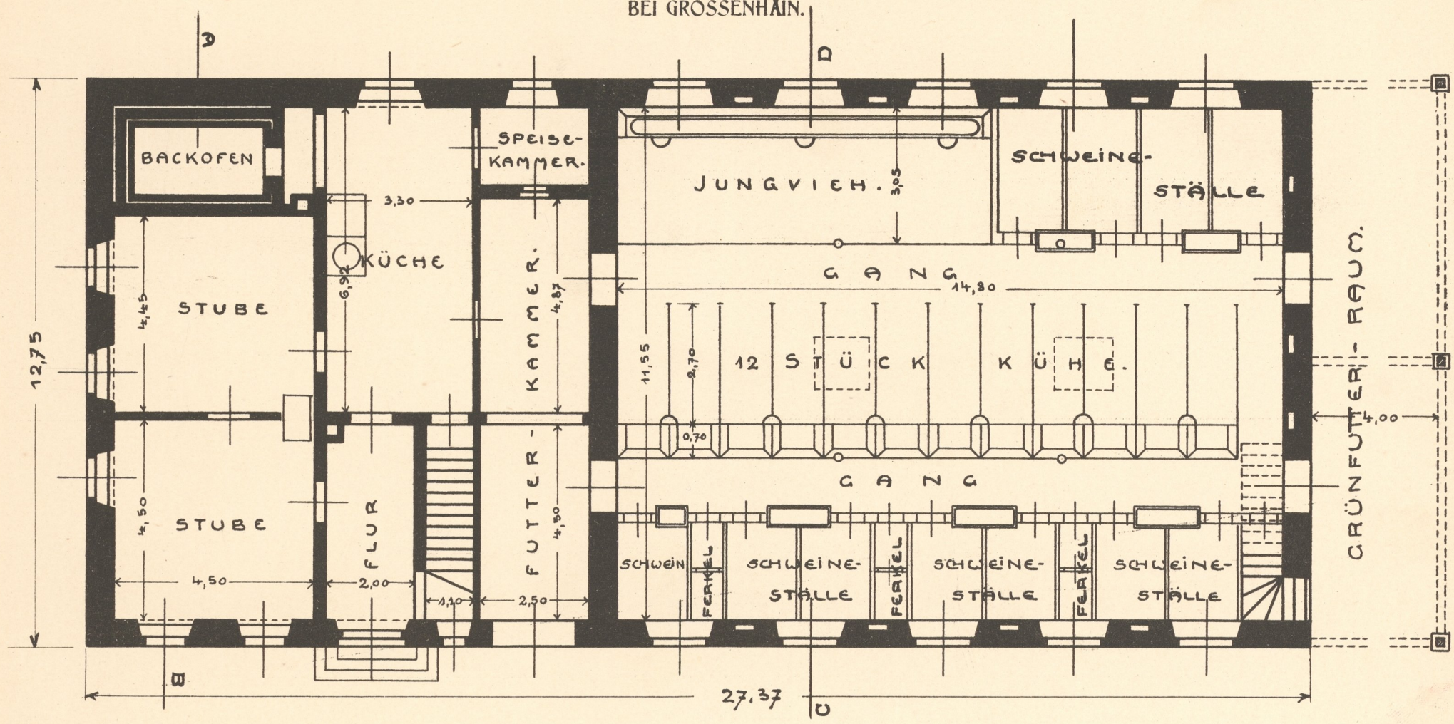
ERDGESCHOSS
