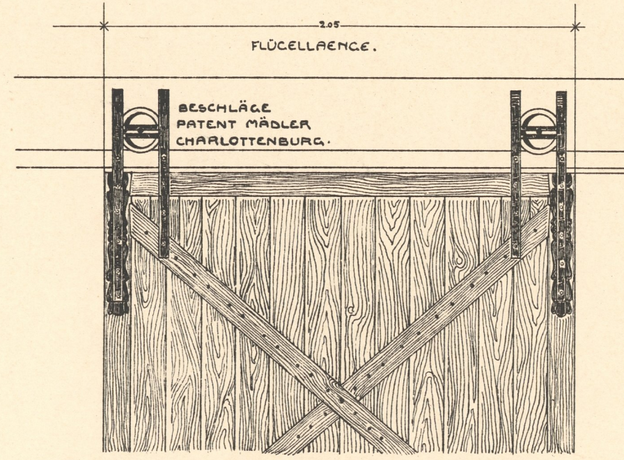
ANSICHT.
