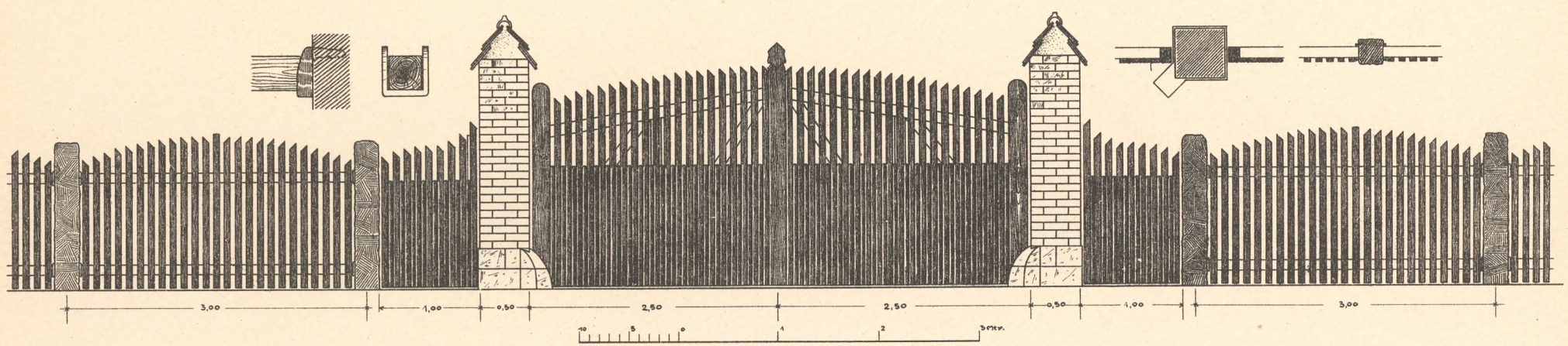
EINFRIEDIGUNG AN DER STRASSE NACH ZWICKAU
