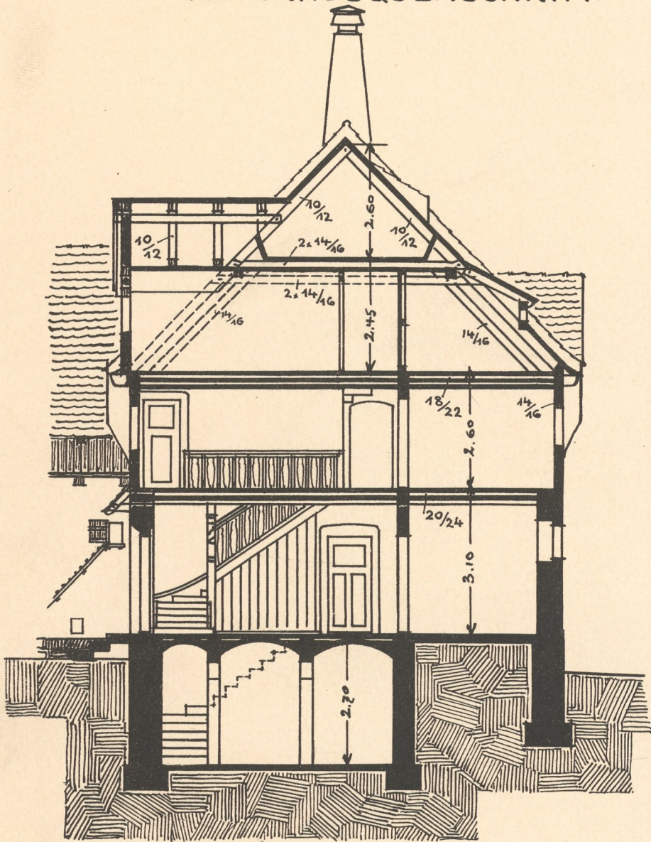
WOHNHAUSQUERSCHNITT.
