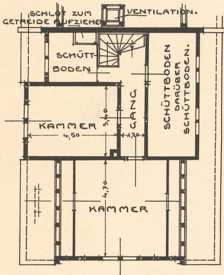
DACHGESCHOSS.
