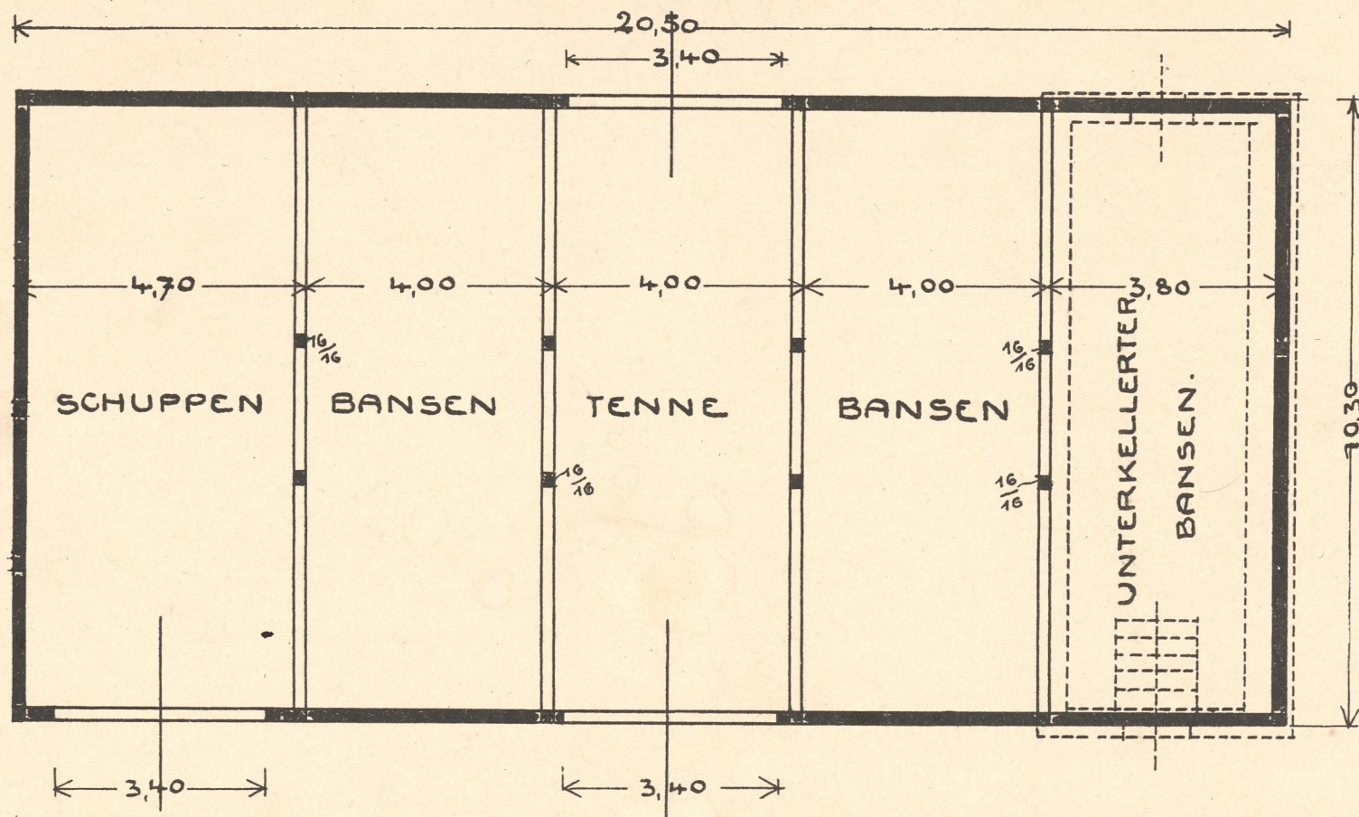
GRUNDRISS.
