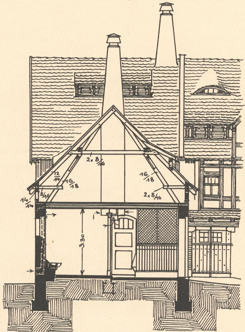
STALLQUERSCHNITT.
