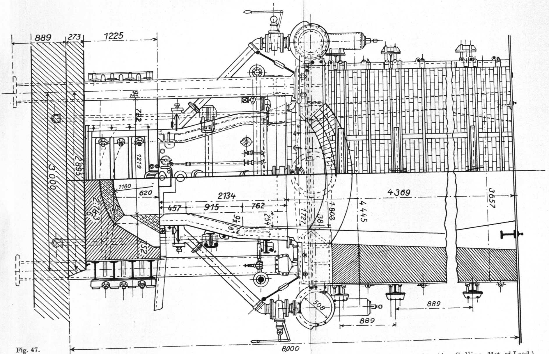
Fig. 46 und 47. Bleischmelzofen (Laurium) mit automatischem Stich in 2 aufeinander senkrechten Schnitten und in Aufsicht. (Aus Collins, Met. of Lead.) Maße in mm.
