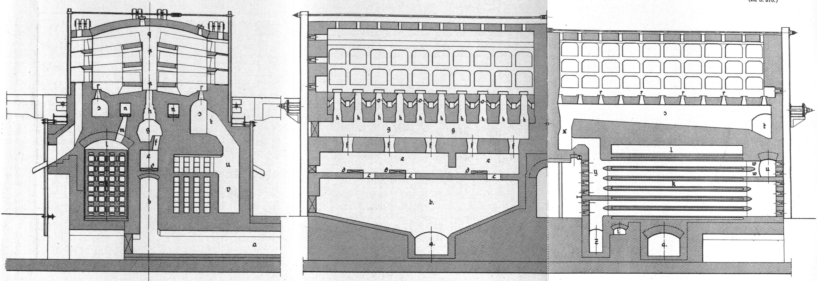
Fig. 122. Rekuperativofen mit Rekuperatoren Bauart Hecker für 240 Muffeln (Erb.: Bender & Främbs, G.m.b.H., Hagen i. W.). Maßstab 1 : 75.
