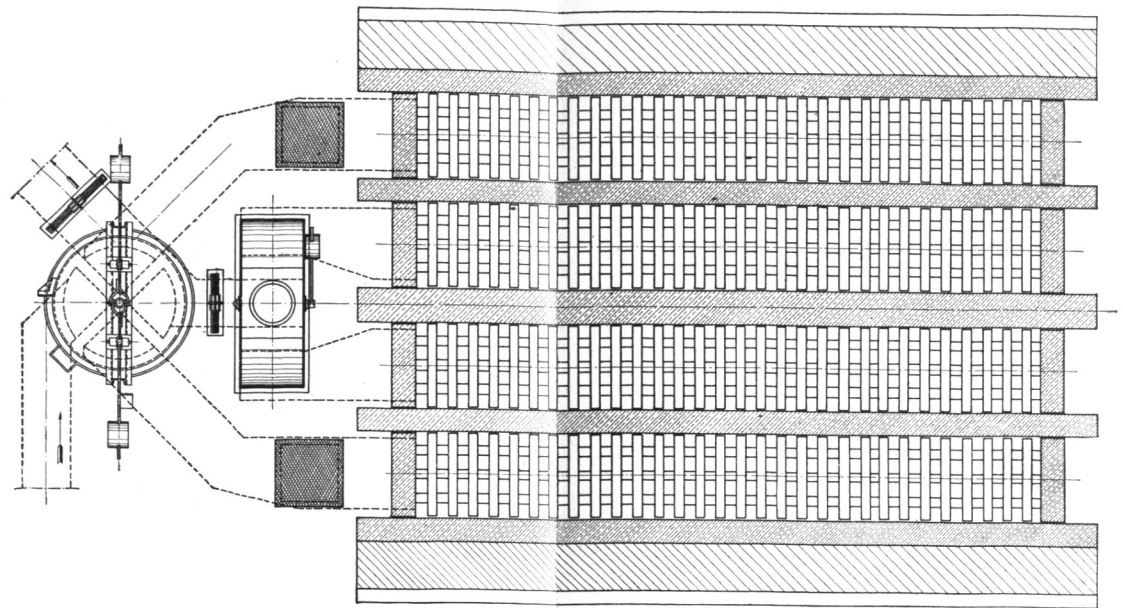
Grundriß
