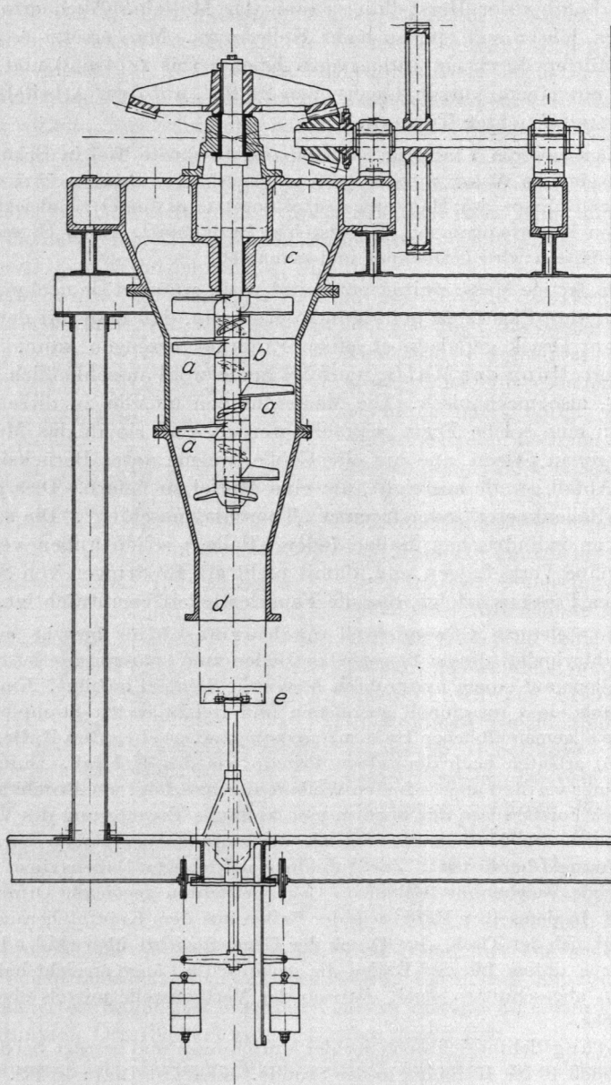
Fig. 106. Ballenpresse der Maschinenbauanstalt C. Mehler, Aachen.
