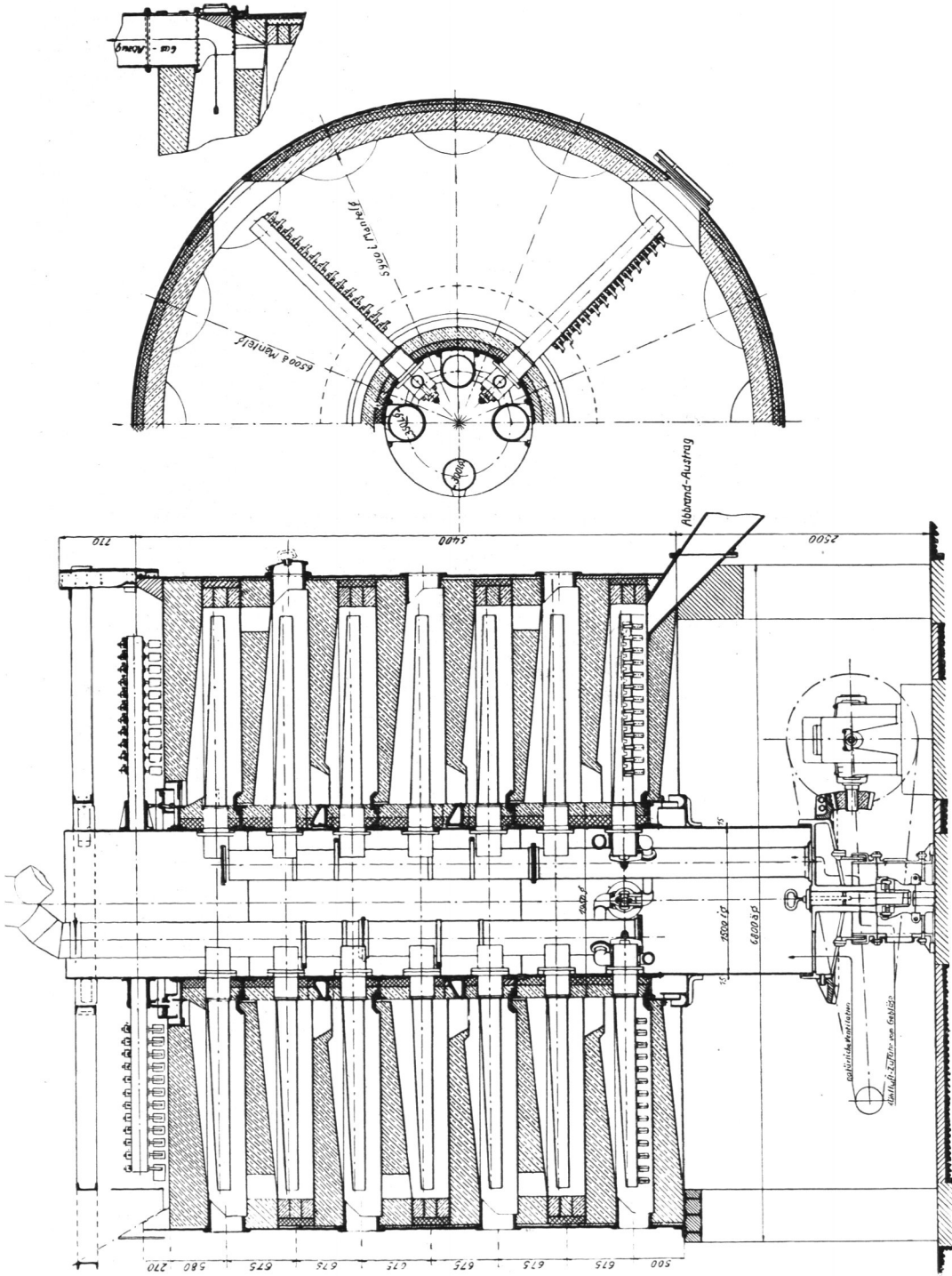
Fig. 99. Vorröstofen der Maschinenbauanstalt Humboldt, Köln-Kalk. 7 Röstherde, 1 Trockenherd. Produktion: 65 bis 75 t. Maße in mm.
