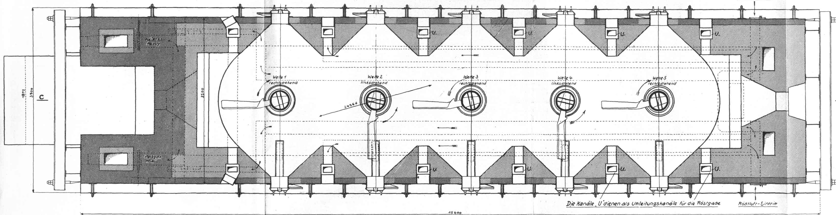
Fig. 97 d Schnitt a-b
