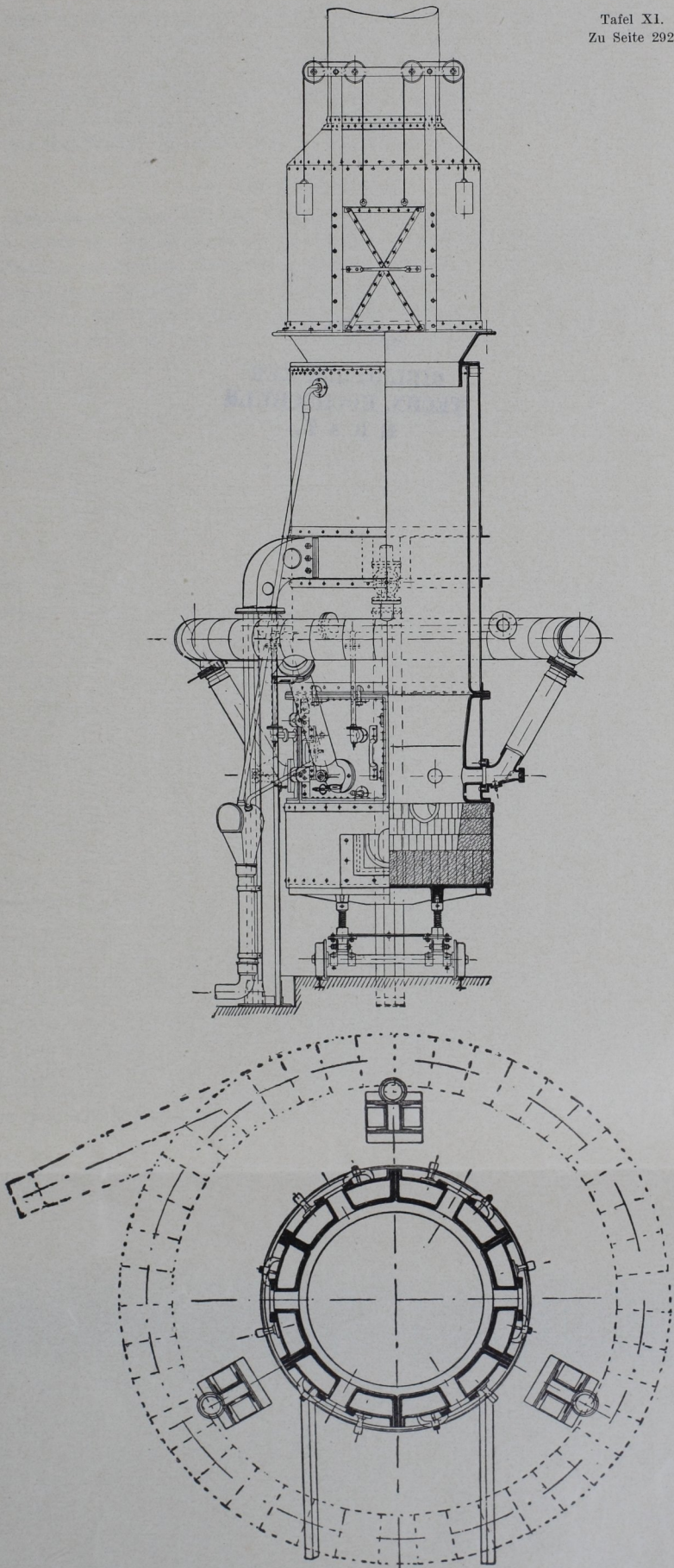
Fig. 116. Kupolofen mit ausfahbarem Tiegel; Bauart Krupp, Grusonwerk. (Aus Borchers, Kupfer.)
