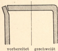
Fig. 464. Stumpfschweißung.
