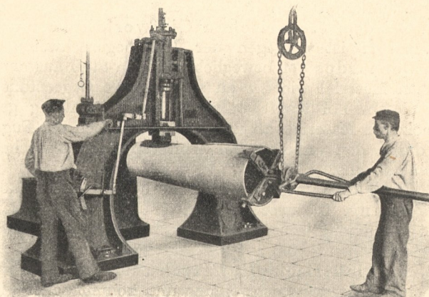
Fig. 467. Schweißhammer.
