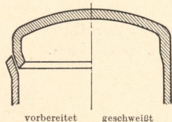
Fig. 465. Überlappte Schweißung.
