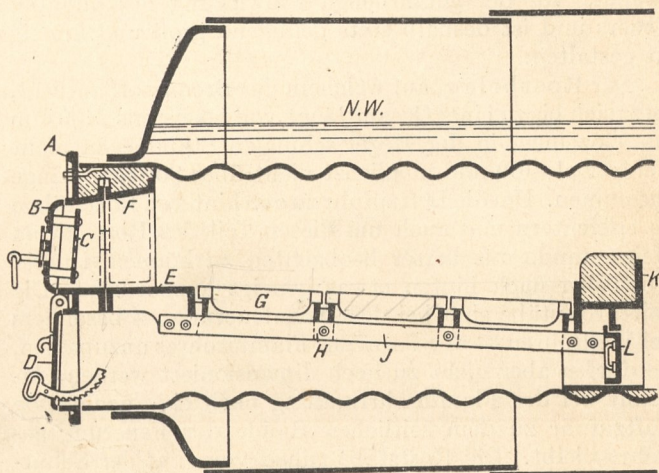
Fig. 205. Planrost-Innenfeuerung.
