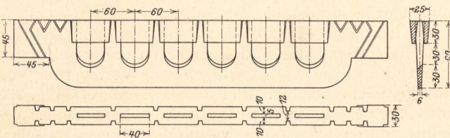
Fig. 212. Geradliniger Roststab mit Aussparungen und durchbrochener Bahn.
