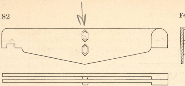
Fig. 210. Mehl-Roststab 1) .
